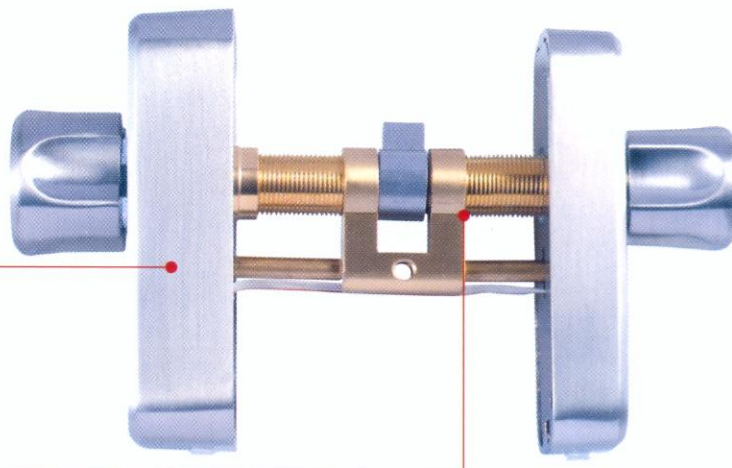
Elektronischer Zylinder ZL: Seitenansicht
